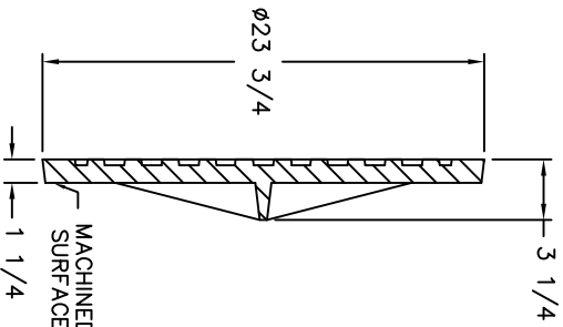
SECTION A-A (E_Cover)
